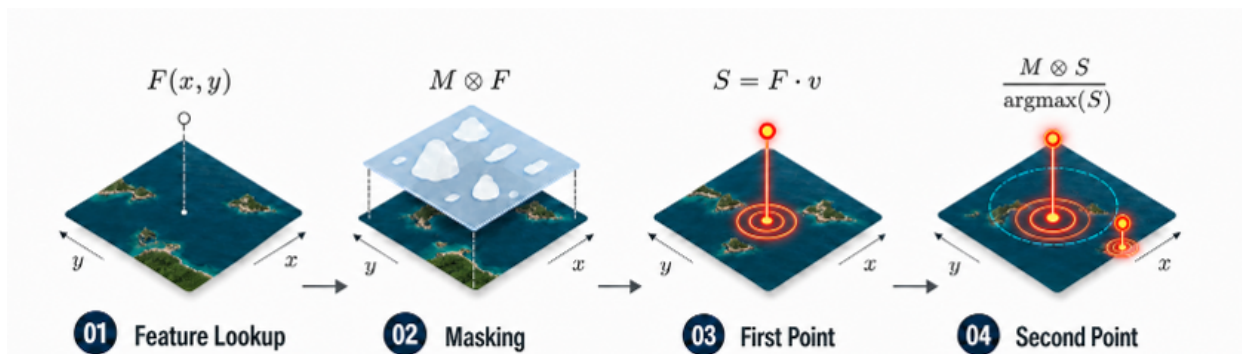
Figure 10: 점수맵 위 픽셀 지목의 네 단계. ① 복호기가 낸 픽셀별 특징 F(x, y) . ② 유효 마스크 M 을 곱해 놓을 수 없는 칸을 차단한다( \text{ifsec:validmask} ). ③ 질의 v 와의 내적으로 점수맵 S = F \cdot v 를 얻고 최대 칸을 첫 점으로 고른다. ④ 첫 점의 특징을 질의에 더해( q \leftarrow q + f_0 ) 같은 절차로 두 번째 점을 고르되, 첫 점과의 간격 상·하한(파선 원)을 마스크에 추가한다. 두 점을 잇는 선분이 그물벽이다.
