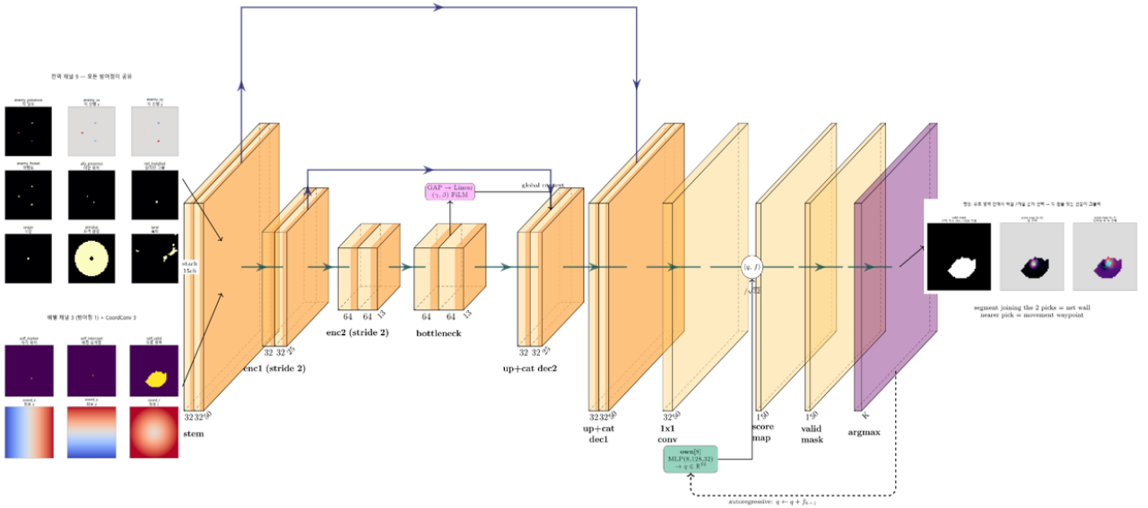
Figure 8: 기동 계층의 텐서 흐름(구현 참조도, 244,389 파라미터, d = 32 , K = 2 ). 왼쪽: 실제 관측 15채널 — 전역 9채널(위)과 방어정별 3채널 + CoordConv 3채널(아래)의 학습된 체크포인트 출력 화면. 가운데: stem → enc1 → enc2(stride 2) → bottleneck → dec2 → dec1의 U-Net. 병목에서 전역 평균 풀링 → 선형층으로 FiLM 계수 (\gamma, \beta) 를 만들어 방어정 자체 상태 \mathbf{o}_p \in \mathbb{R}^8 (MLP 8 \rightarrow 128 \rightarrow 32 )로 조건화한다. 스킵 연결은 위쪽 파란 화살표. 오른쪽: 1 \times 1 합성곱으로 픽셀 특징 f 를 내고, 질의 q 와의 내적 \langle q, f \rangle / \sqrt{d} 로 점수맵을 만든 뒤 유효 마스크를 거쳐 argmax로 K = 2 픽셀을 고른다. 아래 점선은 자기회귀 q \leftarrow q + f_{k-1} — 첫 점의 특징을 질의에 더해 두 번째를 고른다. 본문 Fig. 7는 같은 구조의 개념 일러스트이고, 이 그림은 형상과 조건화 지점을 정확히 적은 판이다.
