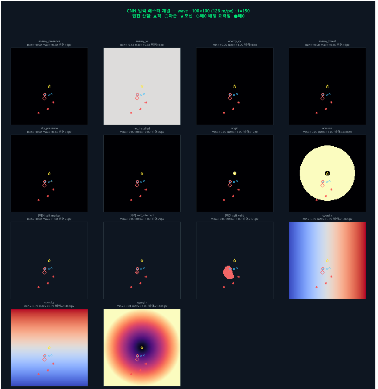
Figure 5: 래스터화된 다채널 관측의 채널별 분해. 전역 채널(적 밀도, 적 진행 x \cdot y , 적 위협도, 아군 위치, 설치된 그물, 원점, 요격 환형), 방어정별 채널(자기 위치, 배경 요격점, 유효 영역), 좌표 채널( x, y, r )이 같은 격자에 정렬된다. 각 패널에 min/max와 비영 픽셀 수를 함께 표시하였다. 이 그림은 시각적 판독을 위해 100 \times 100 (126 m/px)로 렌더하였다 — 본문의 학습·평가 설정은 50 \times 50 (252 m/px)이며 채널 구성과 의미는 동일하다. 육지 채널은 이 장면에 육지가 없어 표시되지 않았다.
